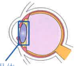
水晶体
